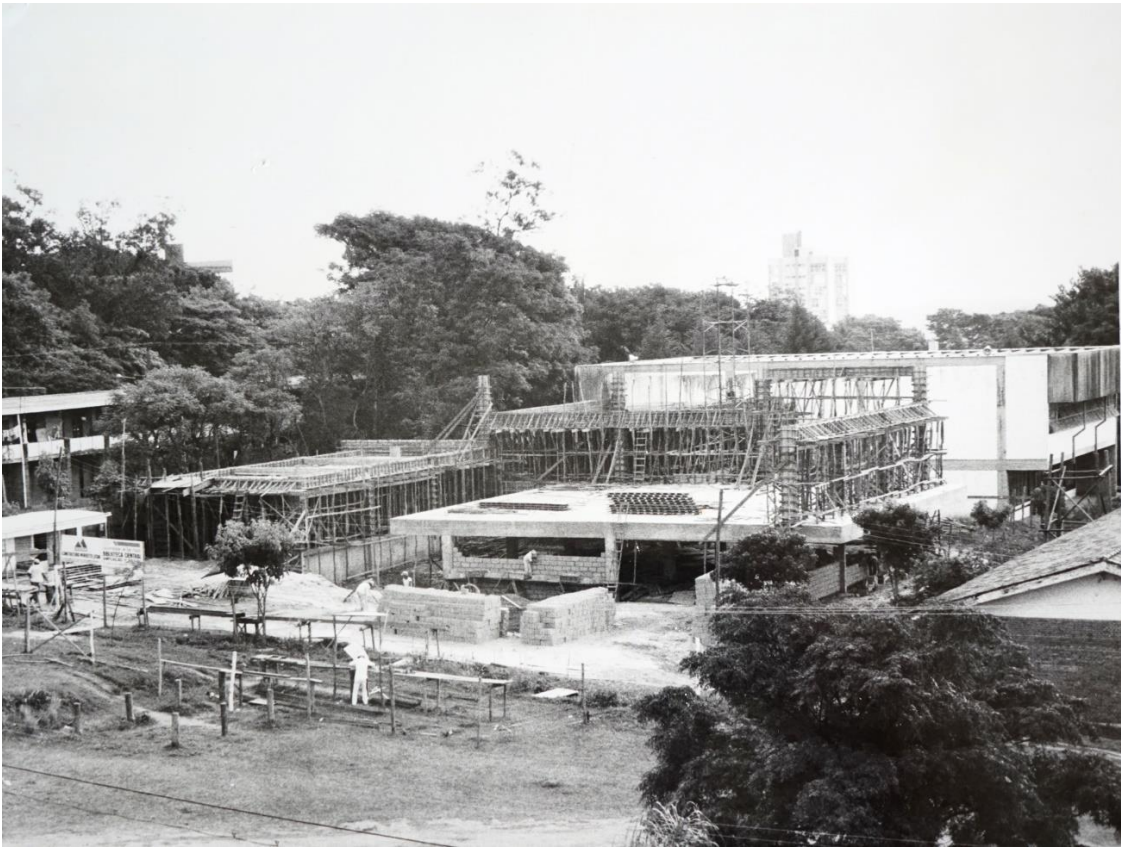
Construção do segundo piso da ampliação da biblioteca central em setembro de 1991. Autor: Calcinha
