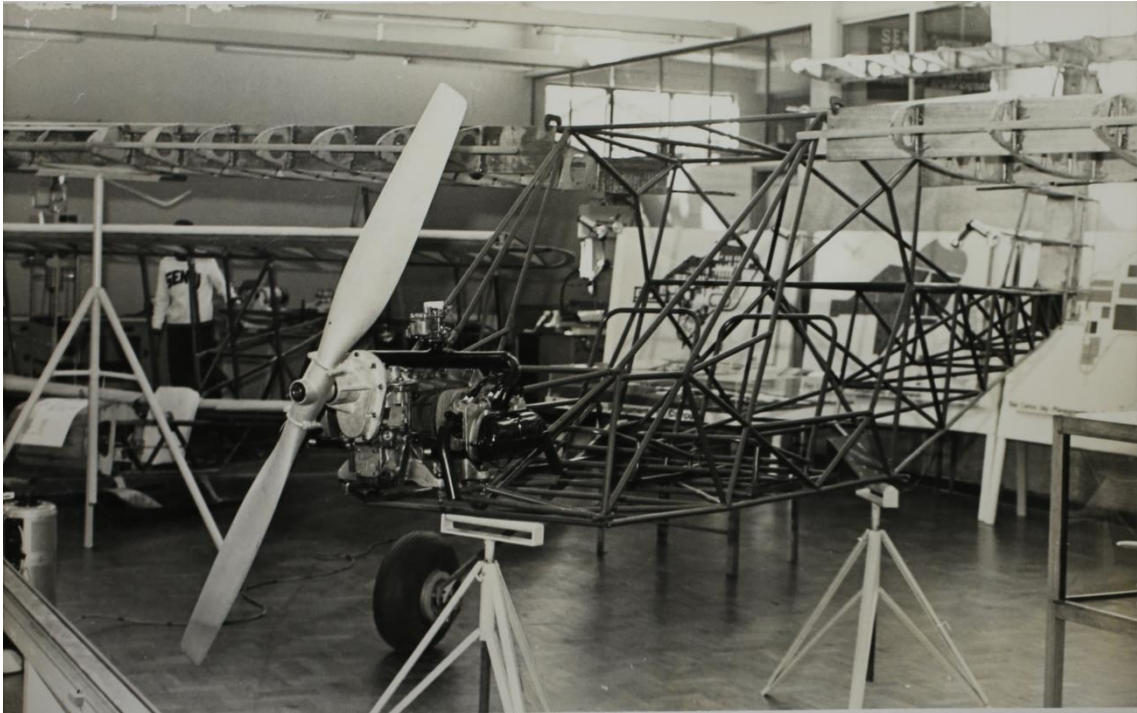
Foto 3 - Fuselagem do protótipo do avião IPAI-26
