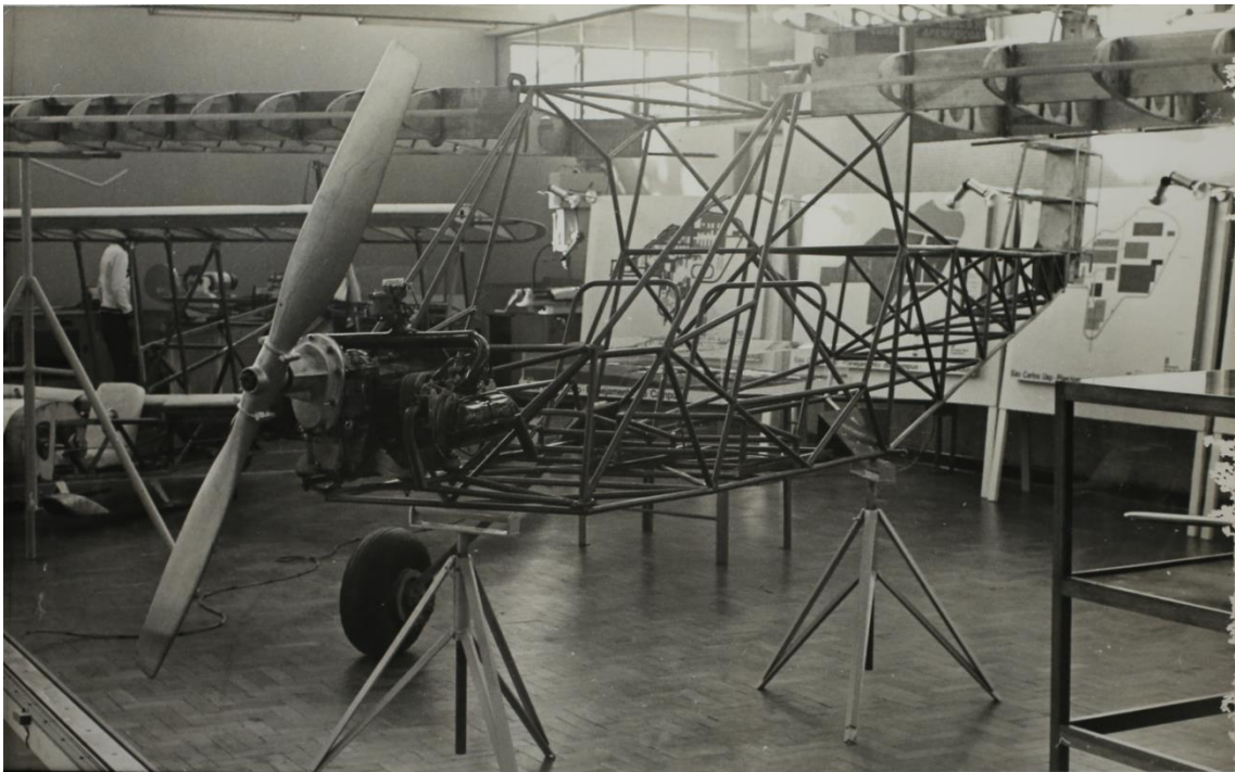
Foto 2 - Fuselagem da estrutura do protótipo do avião IPAI-26 "Tuca" na Mini exposição no SENAI/CIESP, 1973
